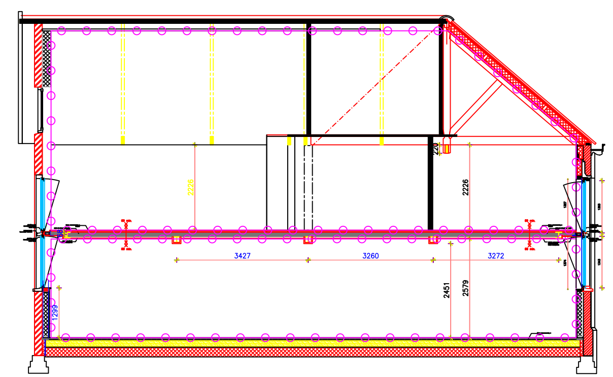
Doorsnede C-C
